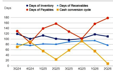
圖 19：經營能力
