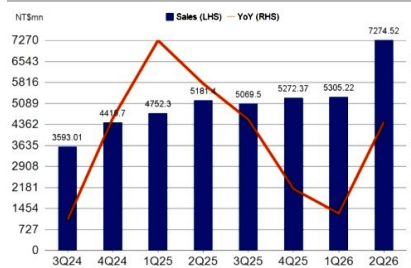
圖 17：營收趨勢
