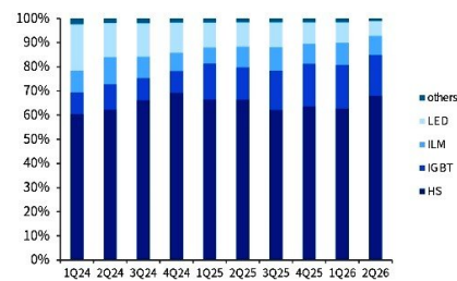
圖 16：營收組成
